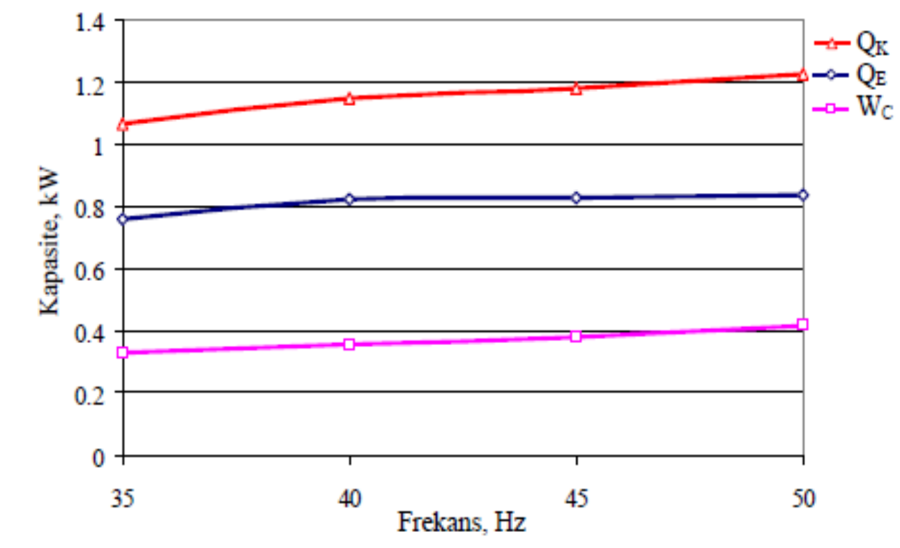
Şekil 2. Kompresör frekansı ile kapasitelerin değişimi
